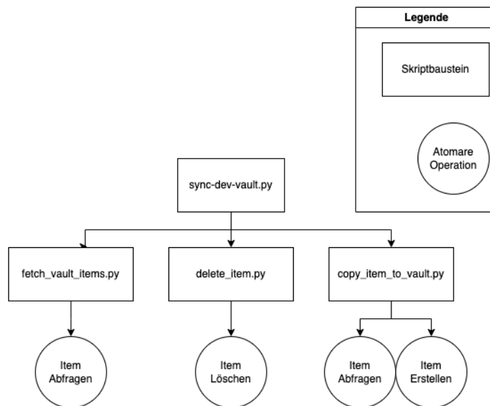
Abbildung 5.: Diagramm: Programmstruktur Secret-Synchronizer
