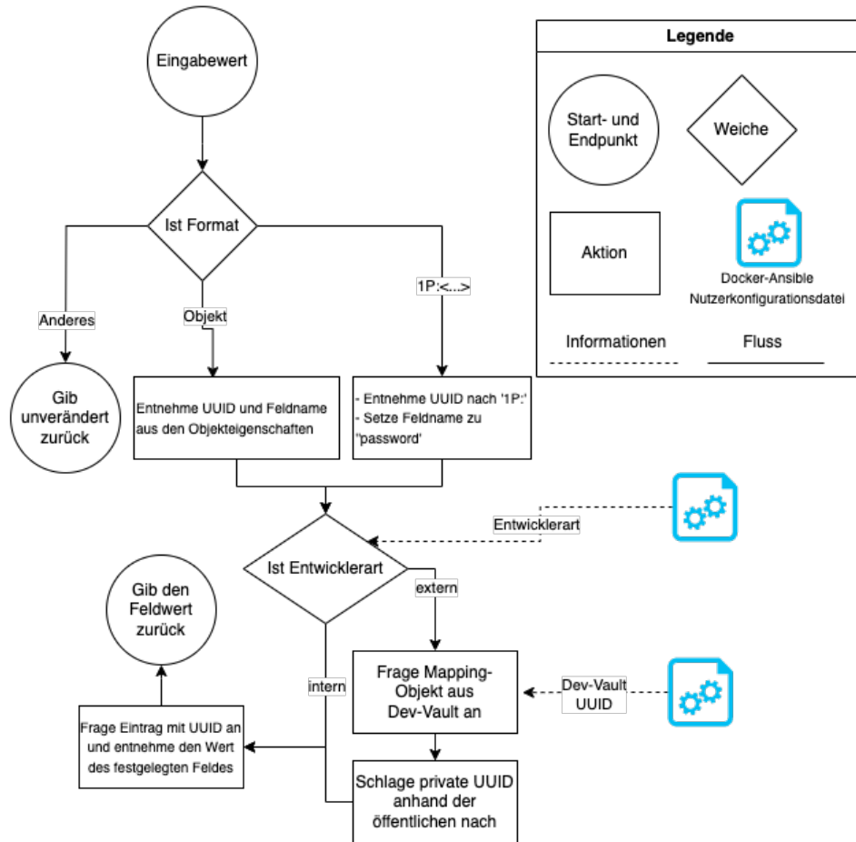
Abbildung 8.: Flussdiagramm: Businesslogik des 1P-Resolver-Filtermoduls
