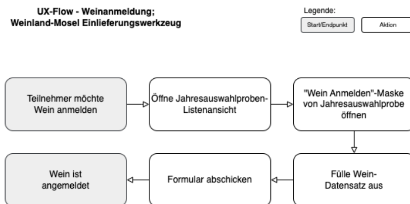
Abbildung 8.: UX-Flow: Weinanmeldung
