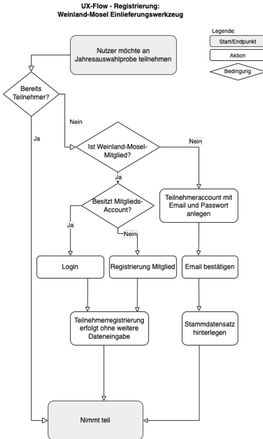
Abbildung 7.: UX-Flow: Registrierung
